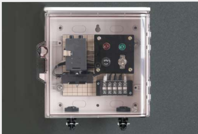
盒子具備 IP44 防水防塵等級
